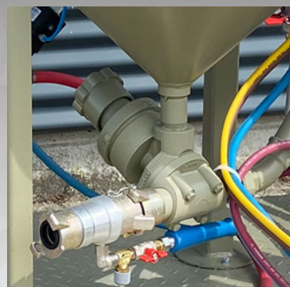
Vandet blandes først med sandet i blæseslangen
