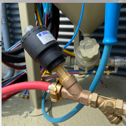
Aktuator der forhindrer vand i at løbe retur i systemet
